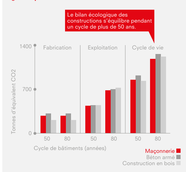
Fig. 2: Empreinte carbone des habitations collectives
