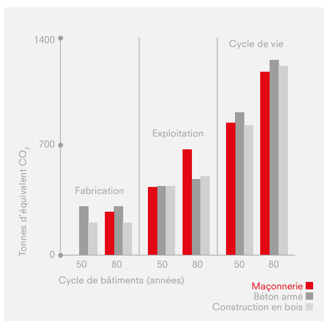
Graphique: Empreinte carbone des habitations collectives. Le bilan écologique des constructions s'équilibre pendant un cycle de plus de 50 ans. (Source: Sebastian Pohl, Robin Schöttner, LCEE Life Cycle Engineering Experts, Mauerwerk, 2019)
